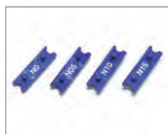
フロントスプリングマウント (MR-03N 0/0.5/1/1.5mm) No.R246-1331B ¥2,860(税込) フロントスプリングにプリロードをかけ られるアルミ製スプリングホルダー。 ナロートレッド用。
