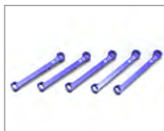
セッティングリンクージ (MR-03/ナロー用-1/0/1/2/3) No.R246-1301 ¥3,080(税込) (MR-03/ワイド用-1/0/1/2/3) No.R246-1302 ¥3,080(税込) MR-03セットアップパーツ、5種類の トア角違いをワンセット。
