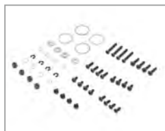
リビルトセット No.R246-1363 ¥550(税込) R246製のMINI-Z用アルミモーター マウント、ロールダンパーに使用してい るビス、ナット、ワッシャーをひとまとめ にしたスペアパーツ。
