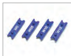
フロントスプリングマウント (MR-03W 0/0.5/1/1.5mm) No.R246-1332B ¥2,860(税込) フロントスプリングにプリロードをかけ られるアルミ製スプリングホルダー。 ワイドトレッド用。
