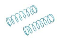
IS106-814 *1100 ビッグダンパースプリング (M/ライトブルー/8-1.4/L=84) Big Shock Spring (M/Light Blue/8-1.4/L=84)
