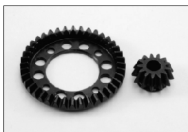
スチールベベルギヤセット(39T) Steel Bevel Gear Set (39T) No.VSW018 ★3990
