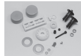
UMW602B ボールデフセット (アルティマ/スコロピオン) Ball Diff. Set (Ultima/Scorpion)
