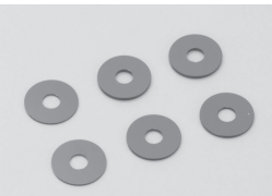
TFW004 ホイールスペーサーセット (4x12x0.5/0.75/1.0/レッド) Wheel Spacer Set (4x12x0.5, 0.75, 1.0/Red)
