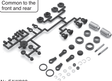
No.FAW302 FZアルミダンパーセット(FZ02/02L/D2) FZ Aluminum Shock Set (FZ02/02L/D2)
