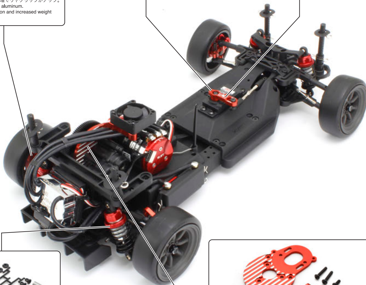
No.FAW310 アジャスタブルアルミサーボホーン(FZD2/17-21/23T) Adjustable Aluminum Servo Horn FZD2/17-21/23T) アルミ製で剛性が向上することで安定したドリフトが可能。 軸間17~21mmで可変 サンワ・KO・ル・マン240Sサーボ用。 Improved rigidity of the aluminum allows for stable drifting. Variable from 17 to 21 mm between the axles (For Sanwa, KO, Le Mans 240S servo).
