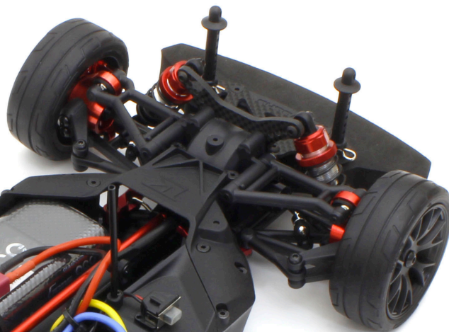
No.FAW223B TCカーボンリヤダンパーステア FZ02 TC Carbon Rear Shock Stay FZ02
