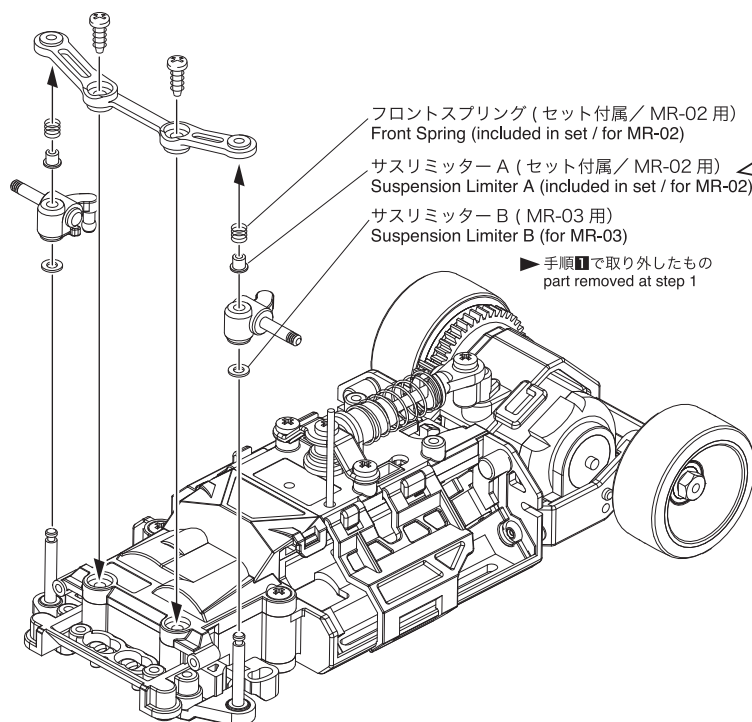
サスリミッター A Suspension Limiter A
