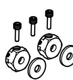
Wide Wheel HexDriver (2+1mm/OPTIMA) ワイドホイールハブセット (2+1mm/2入/オブティマ)
