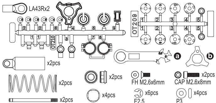
Front Shock Set (Turbo Scorpion) フロントショックセット (ターボスコピオン)
