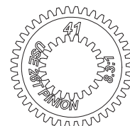
SC225B b x1 Spur Gear 41T スパーギヤ41T
