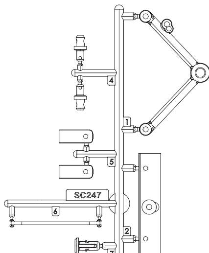
SCB004-01 x1 Light Guard Set (Tomahawk) ライトガードセット (トマホーク)
