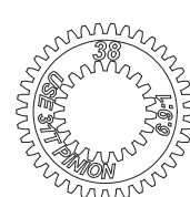
SC225B c x1 Spur Gear 38T スパーギヤ38T
