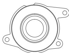
SC205c x1 Side Cover サイドカバー
