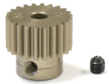
W0122V *500 ベルベットコートピニオンギヤ (22T-48P) Velvet Coating Pinion Gear (22T-48P)
