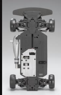
高い放熱効果を発揮するアルミニウムインジェクションキャストと、丈夫な樹脂製バスタブを組み合わせたハイブリッドシャーシを新開発。軽量化とシャーシ全体の剛性化を実現。
