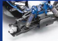
フロントにはユニバーサルジョイントを装備。また、アッパーアームとタイロッドはターンバックル式を採用。エキスパートも納得の装備。
